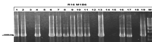
Слика 1 Резултат од електрофорезата во 1% агарозен гел на PCR
